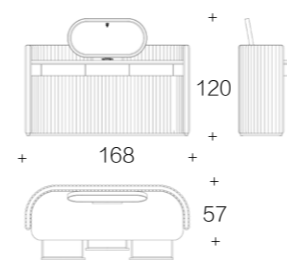
D-VIZT-04 | 妆台 1680*570*1200
