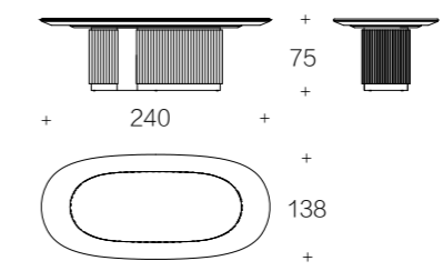
D-CCCZ-04 | 餐桌 2400*1380*750
