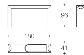
D-VIGT-02 | 玄关台 1800*410*960
