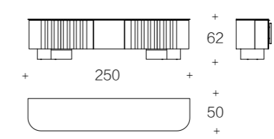
WH309H12 | 电视柜 2500*500*620
