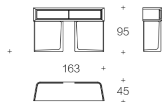
D-VIGT-01 | 玄关 1500*400*930
